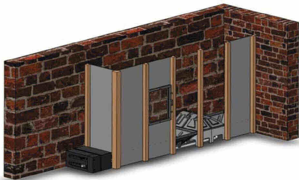
Solución tipo 3 UniWoks®RAPS + 2 BLIND-UniWok®. Salida de pellets por parte estrecha. Centralita automática externa
