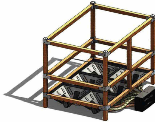
Almacenamiento con saco téxtil y estructura de madera
