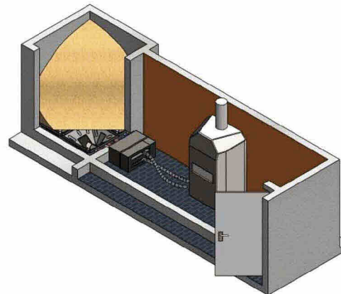
Esquema de instalación con caldera
